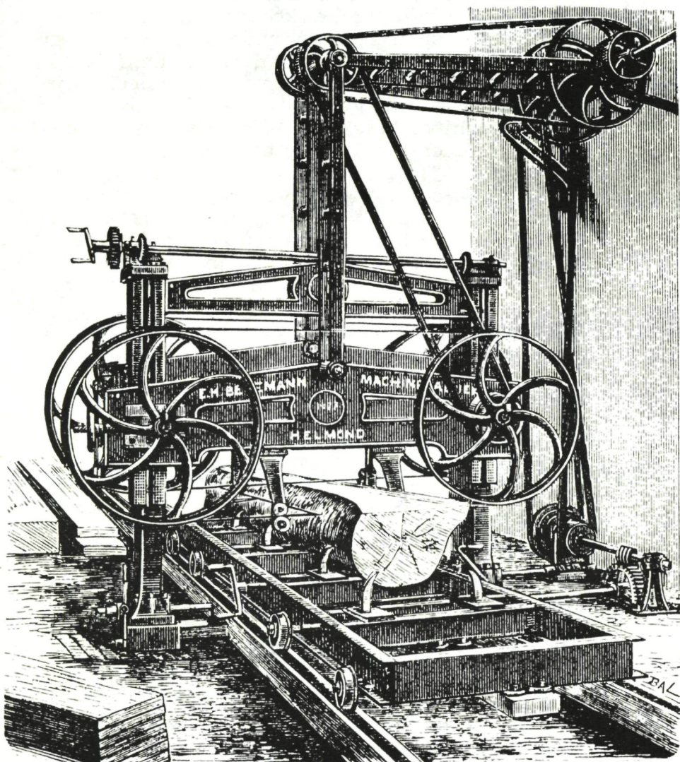
Een bij Begemann geproduceerde horizontale lintzaag om hout te zagen. (Afgebeeld bij: R. Witte, Dubbele horizontale lintzaag. In: Tijdschr. Mij. t.b.v. Nijverh., 1879, blz. 438-444.)
